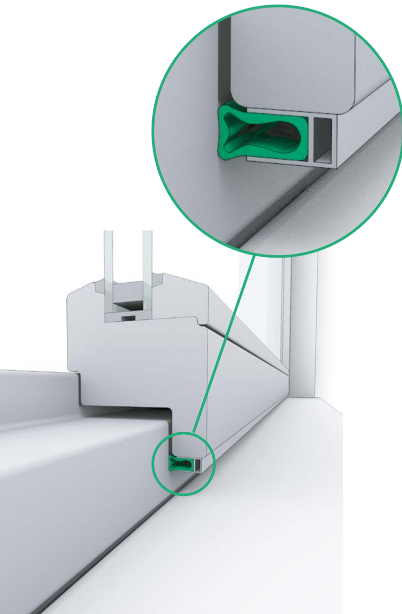
Abb. 7.10: Elastische Dichtungsprofile, eingenutet oder in aufgesetzten Metallprofilen
