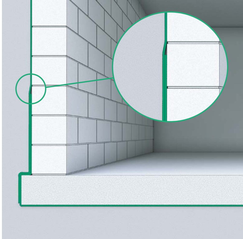
Abb. 7.2: Außenseitige Abdichtung mit Dichtungsbahnen unter der Fundamentplatte (Neubauten)
