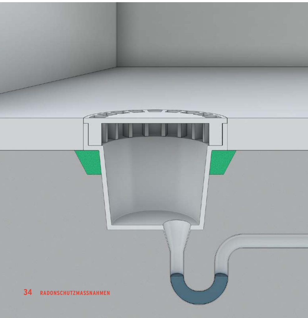
Abb. 7.7: Abdichten eines Bodenablaufs
