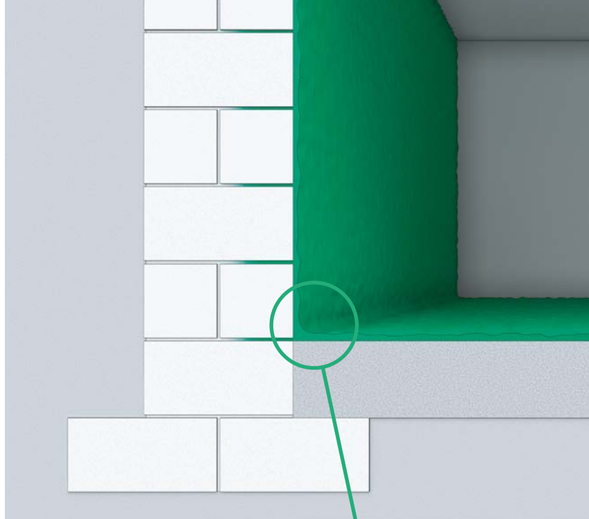
Abb. 7.5: Beschichtungen mit Dichtungsschlämmen und Anstrichen
