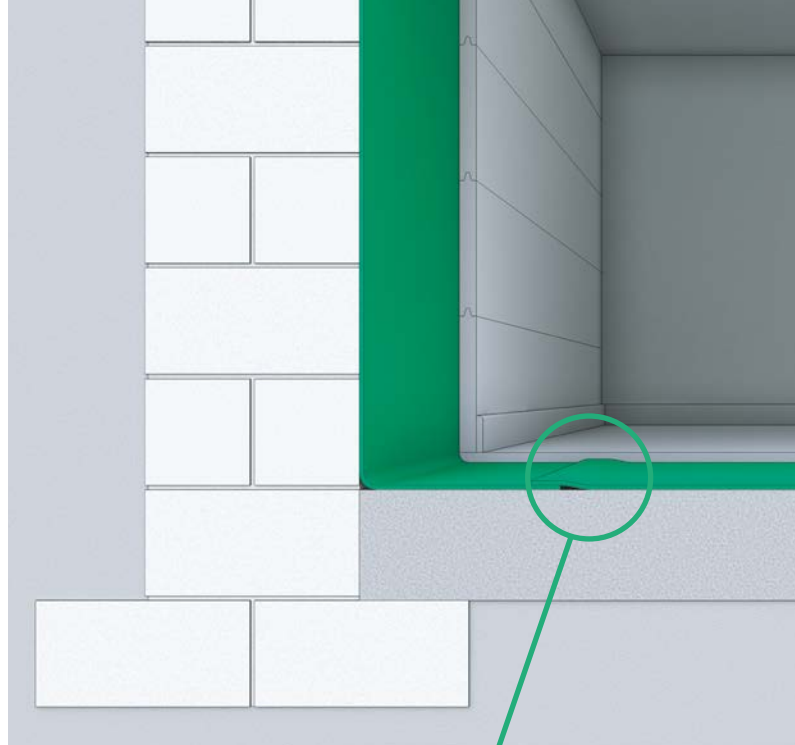
Abb. 7.3: Raumseitige Abdichtung mit Dichtungsbahnen
