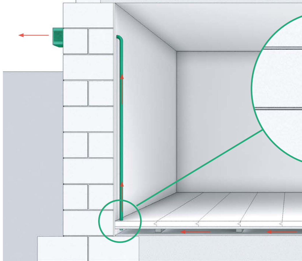
Abb. 7.21: Entlüftung von bestehenden Hohlräumen
