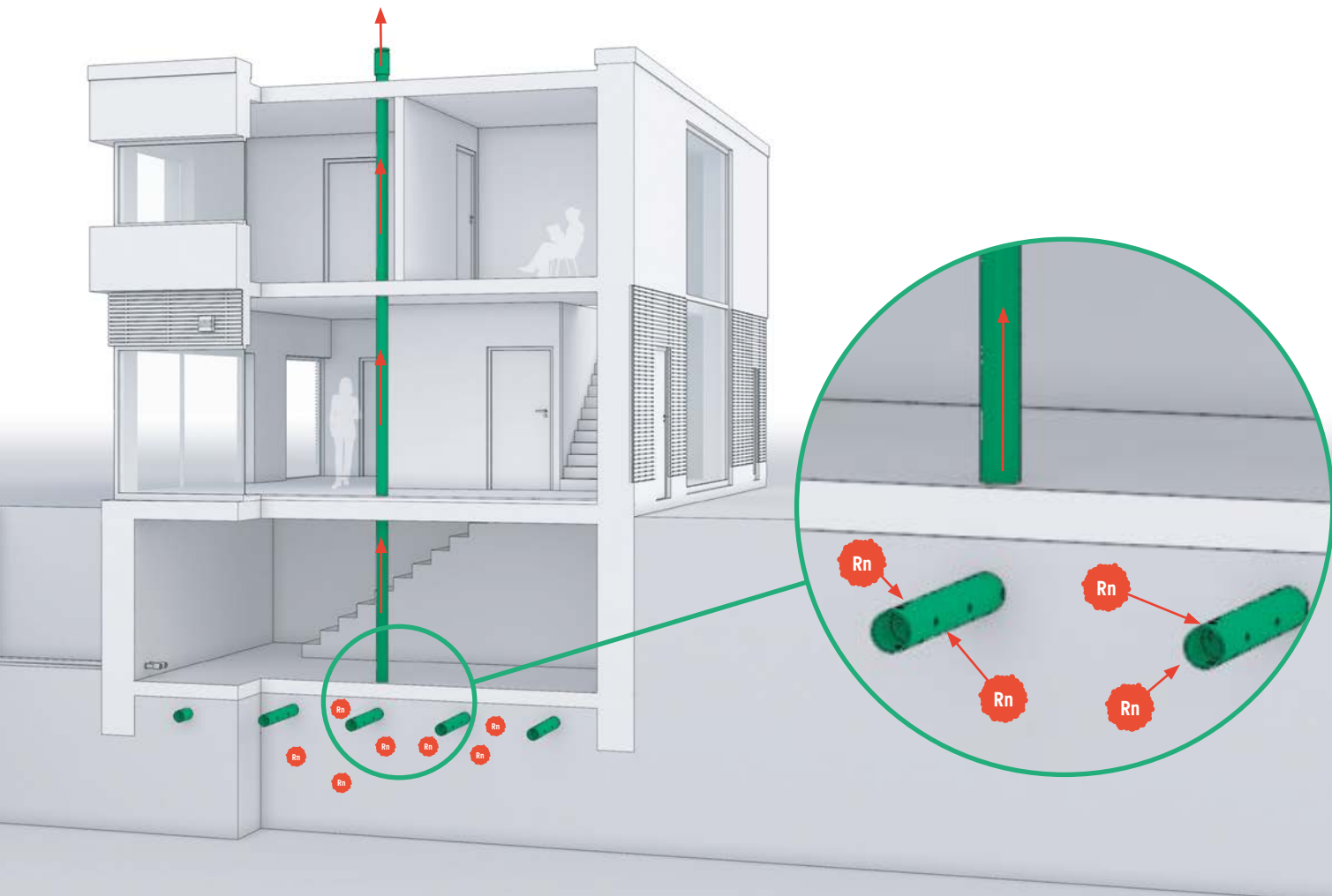
Abb. 7.17: Bodenentlüftung unter der Gebäudesohle mittels Drainagesystem
