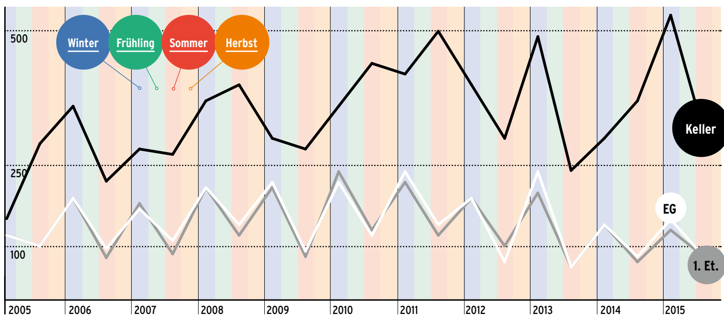
Abb. 6.2: Jahreszeitliche Variation der Radonmittelwerte
