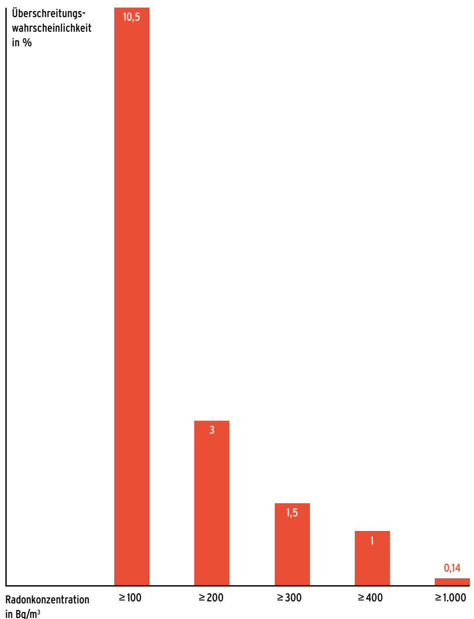
Abb. 4.2: Radonkonzentrationen in Bq/m 3 in Aufenthaltsräumen im Erdgeschoss von Ein- und Zweifamilienhäusern (Quelle: Untersuchung des BfS [16])
