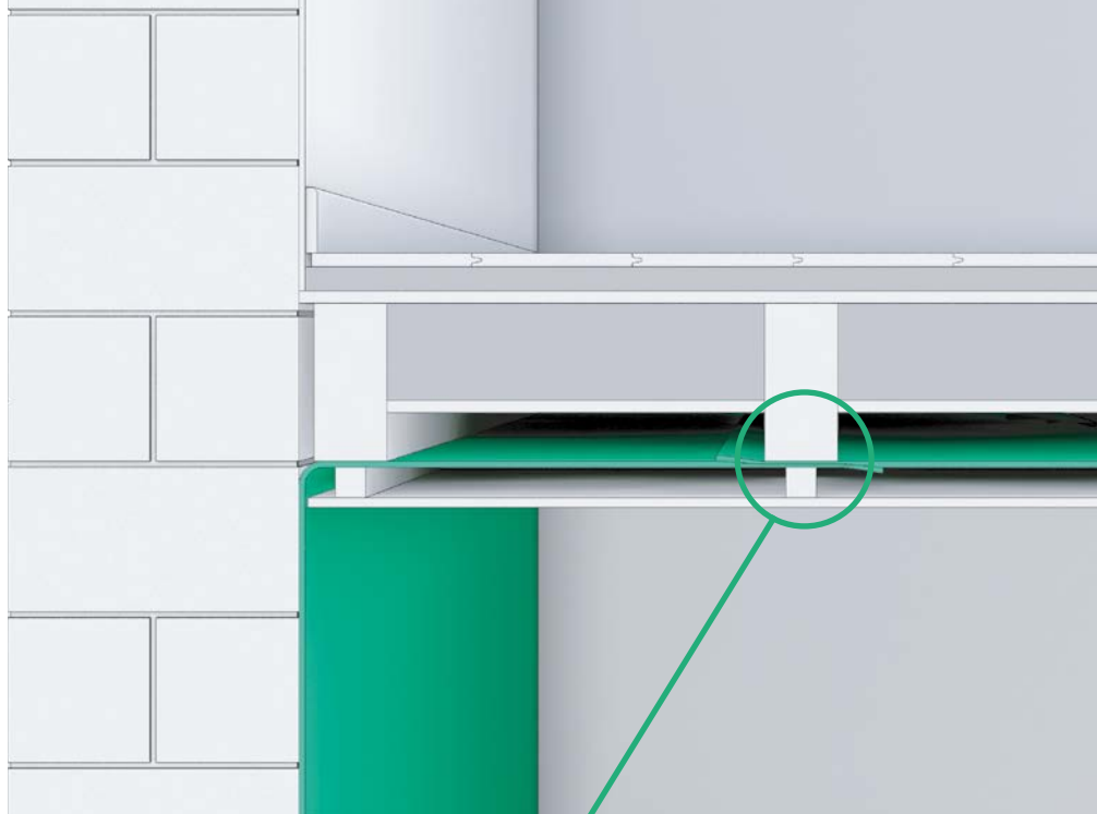
Abb. 7.8: Anschluss Deckenabdichtung
