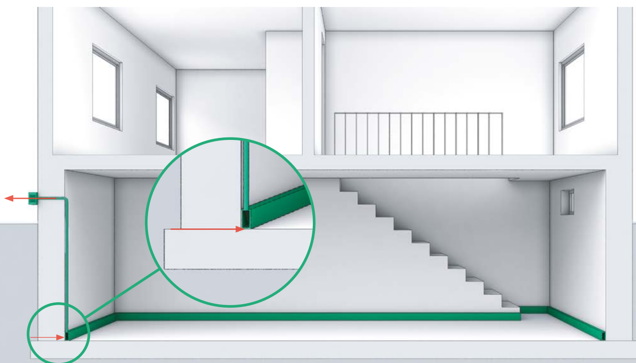
Abb. 7.19: Unterdruckerzeugung unter der Bodenplatte durch Absaugkanal entlang der Bodenplattenfuge
