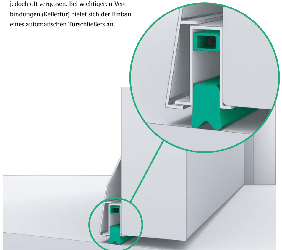
Abb. 7.13: Bewegliche Anpress-Schwellendichtung
