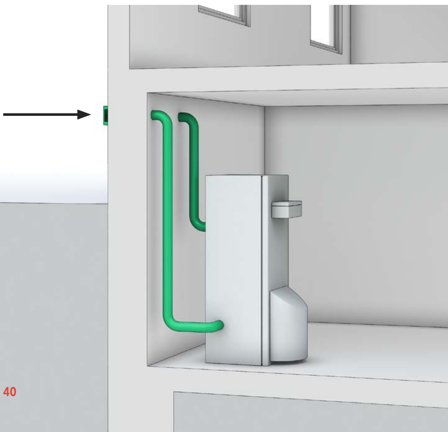
Abb. 7.16: Direkte Außenluftzufuhr zum Brenner
