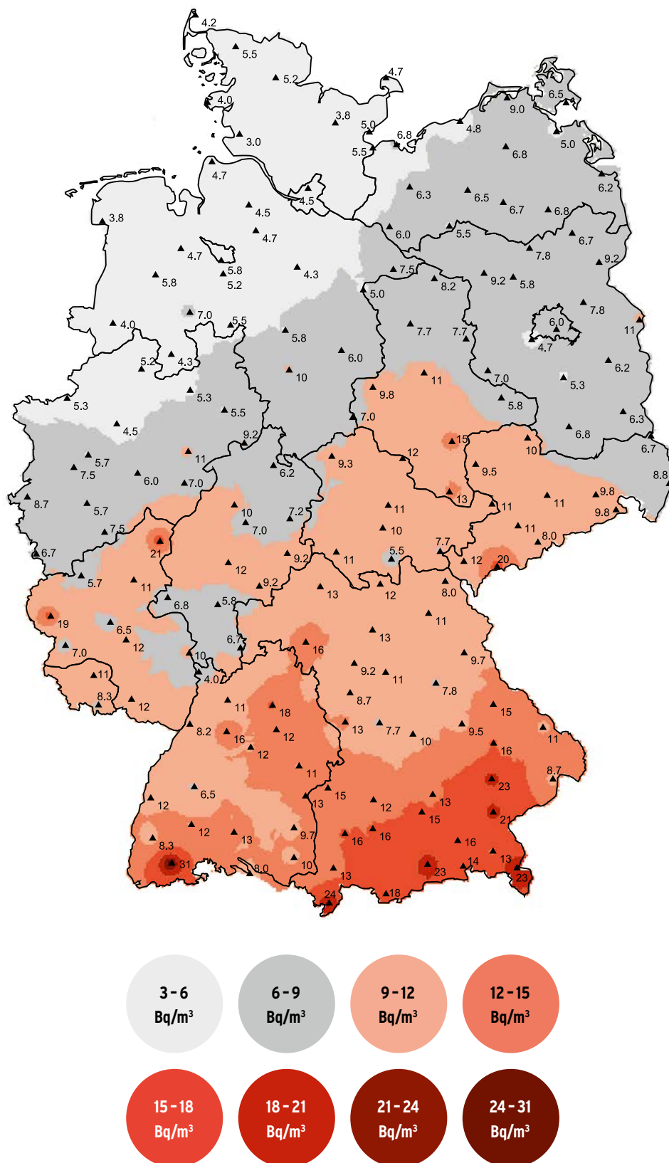
Abb. 3.3: Radon-222-Konzentration in der bodennahen Atmosphäre in Bq/m 3
