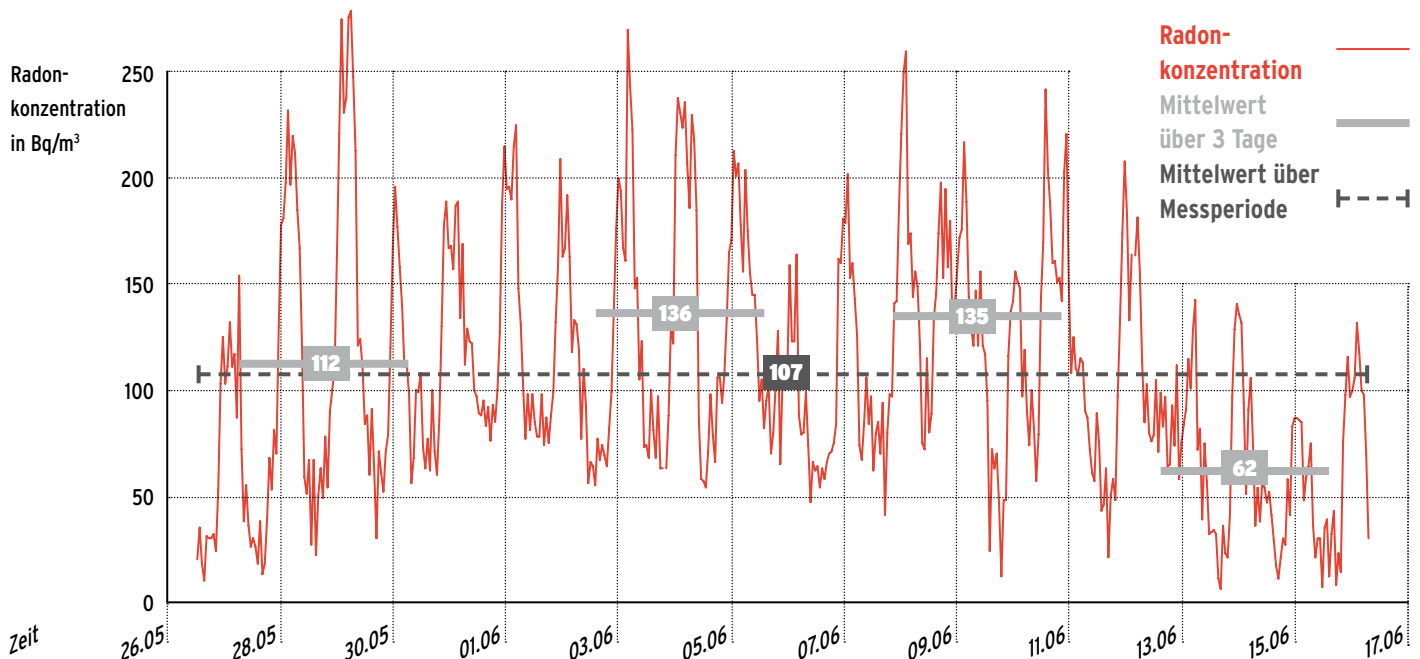
Abb. 6.1: Zeitlicher Verlauf der Radonkonzentration (Beispiel) und Mittelwerte über 3 Tage
