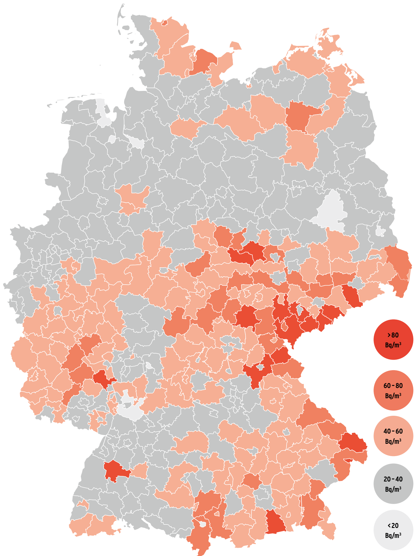
Abb. 4.3: Durchschnittliche Radonkonzentrationen (geometrischer Mittelwert über Landkreise, Stand 2006) in Wohnungen in Deutschland (nach Menzler et al.) [6]
