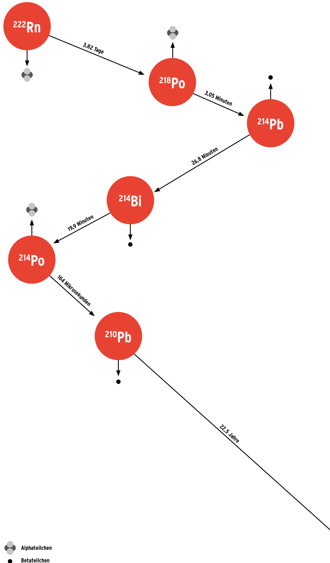
Abb. 1.1: Zerfallsreihe des natürlichen, radioaktiven Isotops Radon-222 mit Halbwertszeiten
