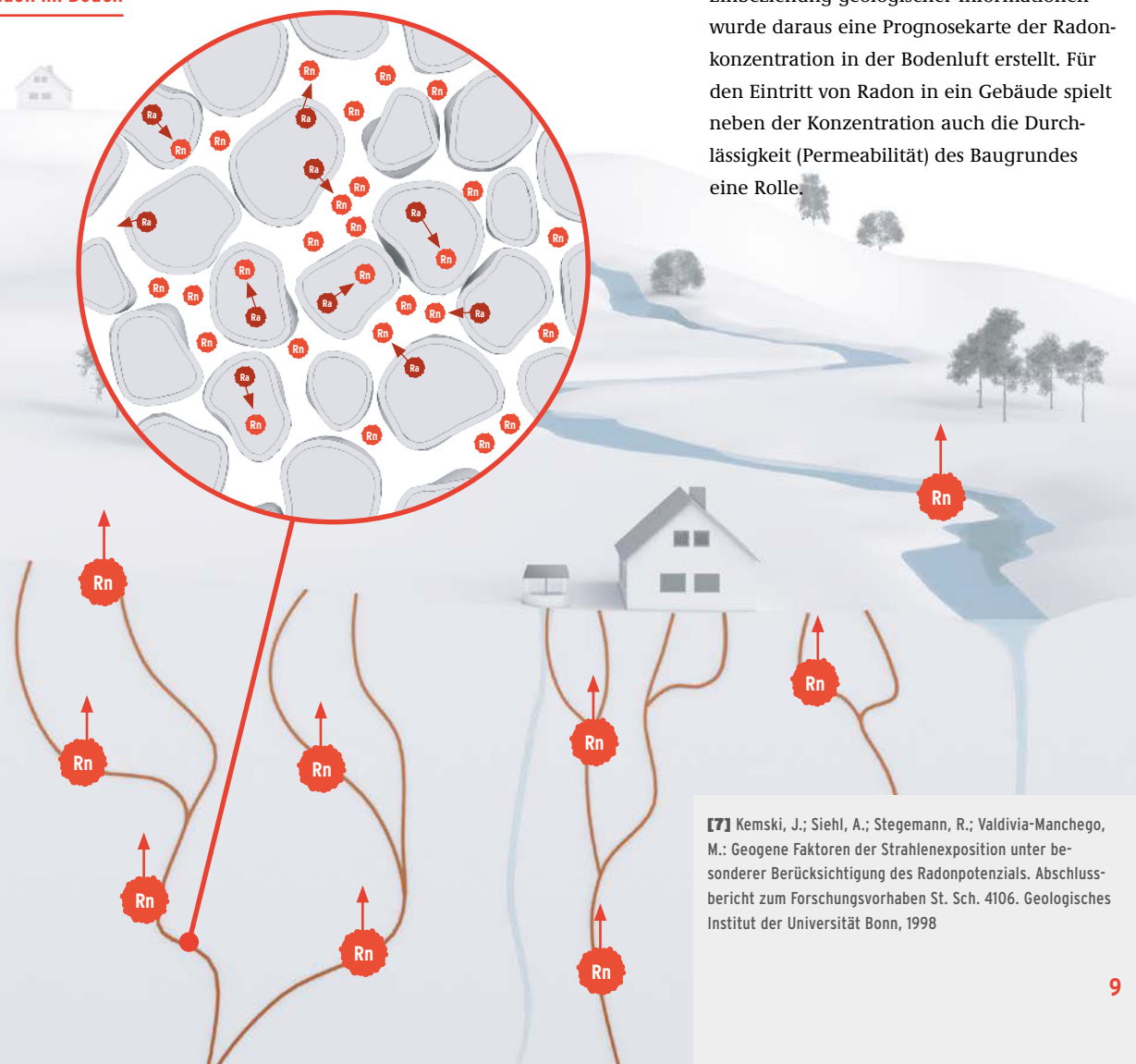
Abb. 3.1: Entstehung und Ausbreitung von Radon im Boden
