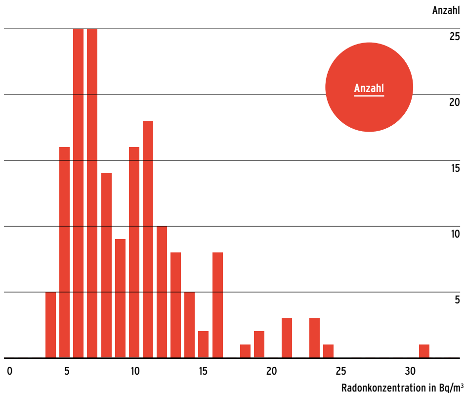
Abb. 3.4: Verteilung der an den Messpunkten vorliegenden Freiluftkonzentrationen (Mittelwert aller Messungen an jedem Standort)
