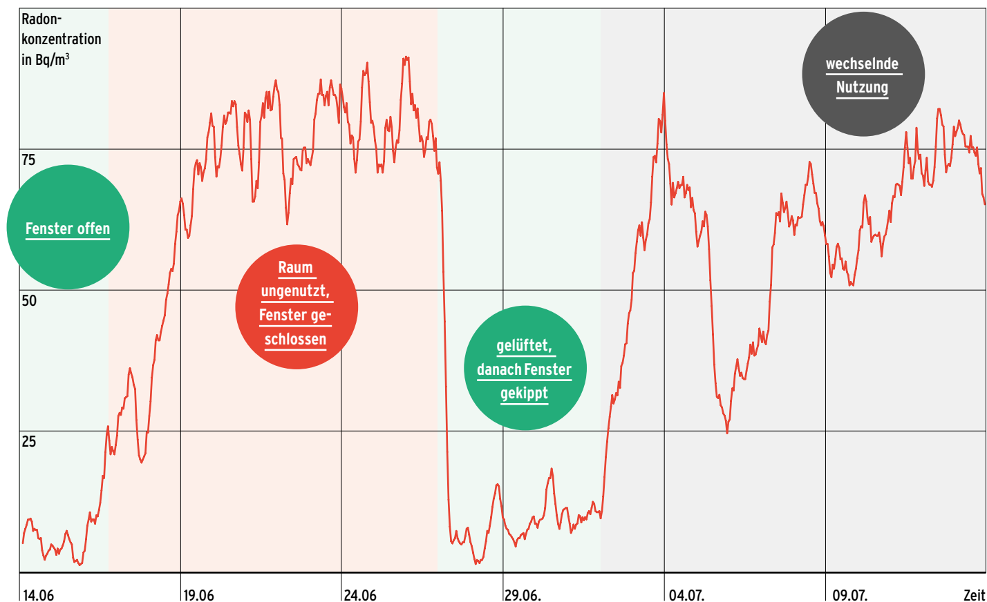
Abb. 4.1: Beispiel für die Auswirkung verschiedener Lüftungen auf die Radonkonzentration in einem Raum
