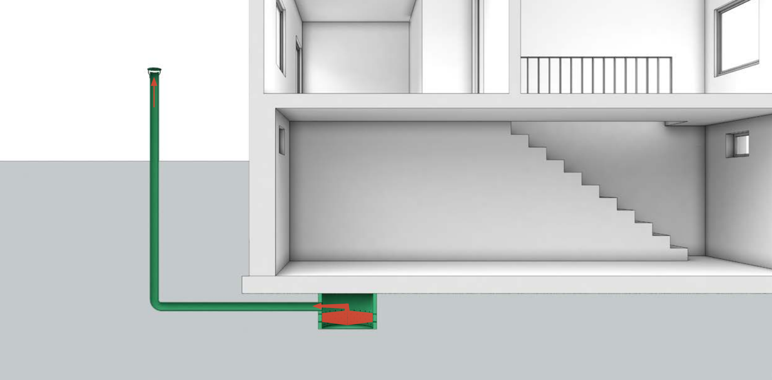
Abb. 7.18: Bodenentlüftung unter der Gebäudesohle mittels Sammelschacht
