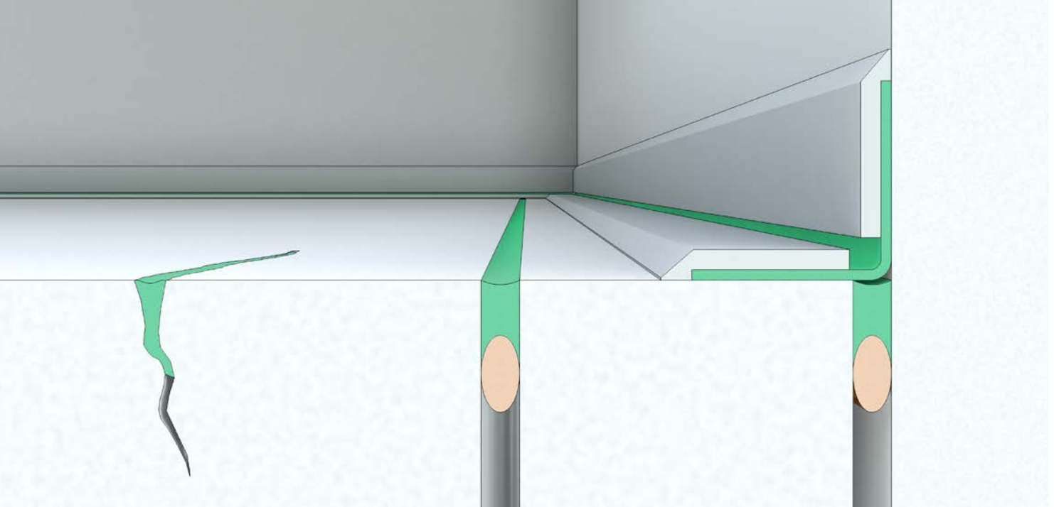
Abb. 7.6: Überbrücken von Dehnungsfugen
