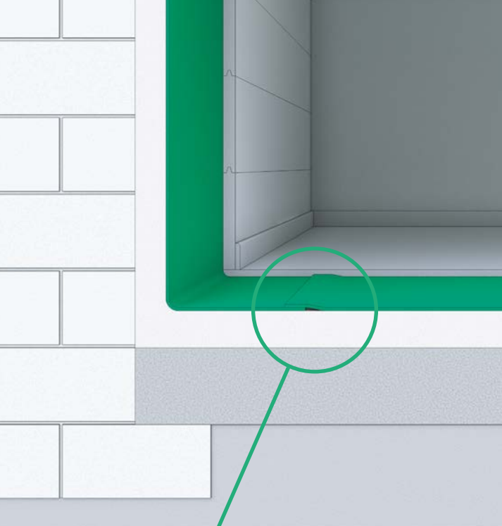
Abb. 7.4: Wärmeisolationsschicht und Radonsperre
