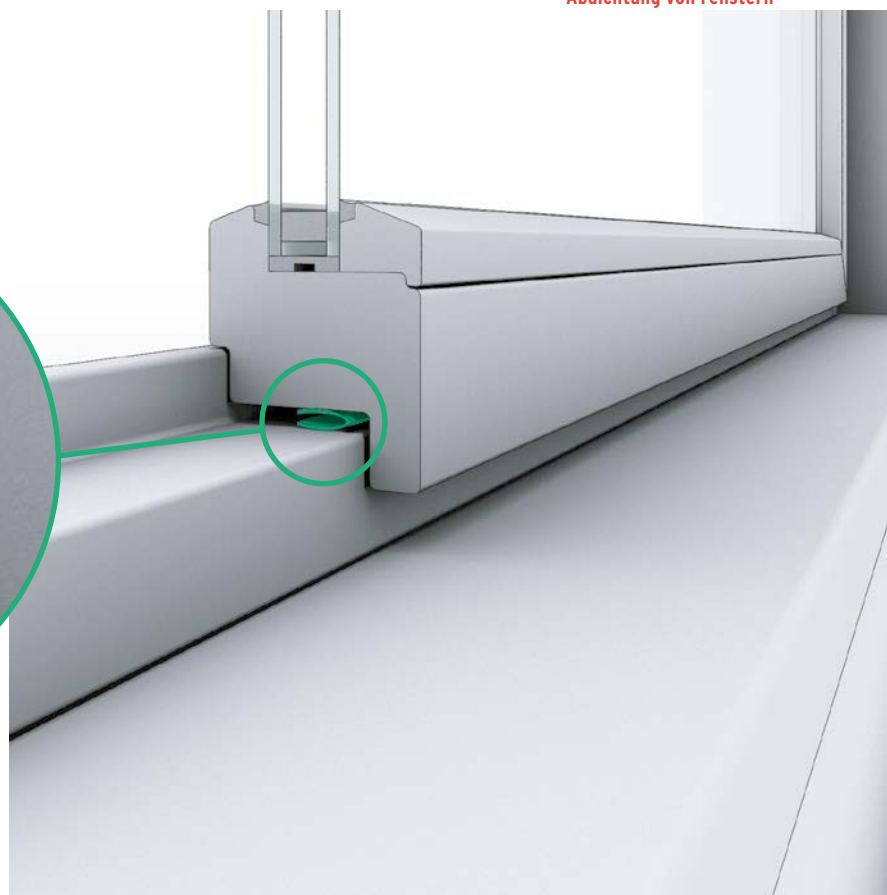
Abb. 7.11: V-Dichtungen für die nachträgliche Abdichtung von Fenstern
