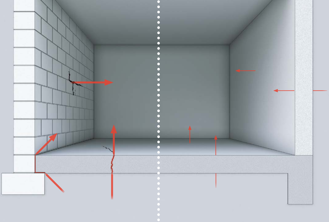
Abb. 7.1: Eindringen von radonhaltiger Bodenluft durch Leckstellen (links) und Diffusion von Radon durch Bauteile hindurch (rechts)
